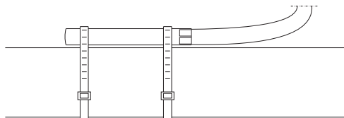
Rys. 7 Sposób montażu czujnika do rury
