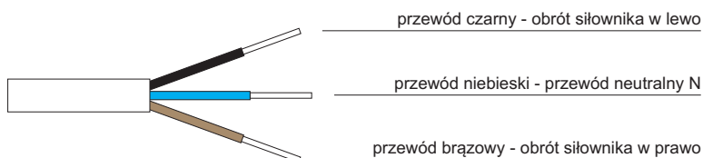
Rys. 5 Opis żył przewodu zasilającego siłownik zaworu 3 lub 4 drog. ~230 V
