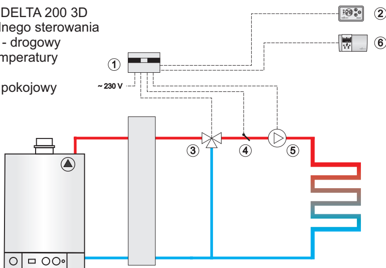
Rys.3 Podłączenie regulatora do instalacji ogrzewania podłogowego z kotłem gazowym i sprzęgłem hydraulicznym
