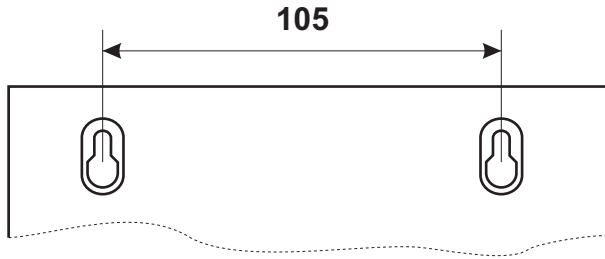
Rys. 10 Rozstaw otworów montażowych
