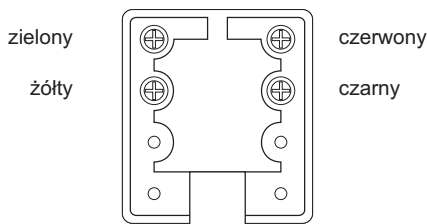
Rys. 9 Rozmieszczenie złącz w puszcze gniazda telefonicznego
