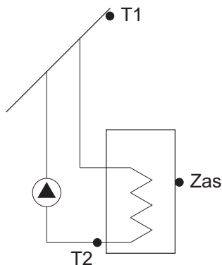
Rys. 5 Schemat montażu czujników - opcja T2 .
