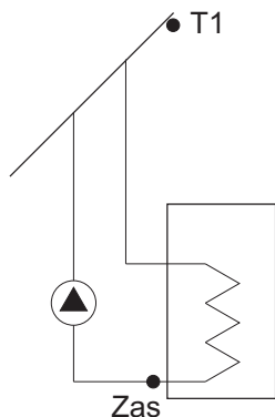
Rys. 4 Schemat montażu czujników - opcja Zas .
