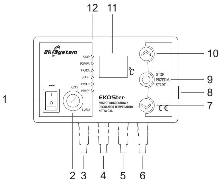
Rys. 2 Elementy regulatora
