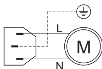
Rys. 1 Schemat podłączenia przewodu do pompy lub wentylatora
