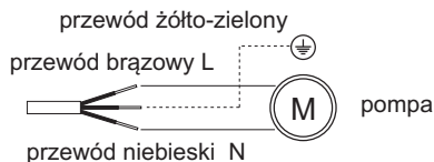
Rys. 6 Schemat podłączenia przewodu do pompy
