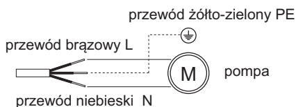
Rys. 4 Schemat podłączenia przewodu do pompy
