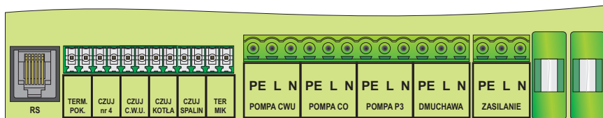
Rys. 8 Opis wyprowadzeń przyłączy sterownika.
