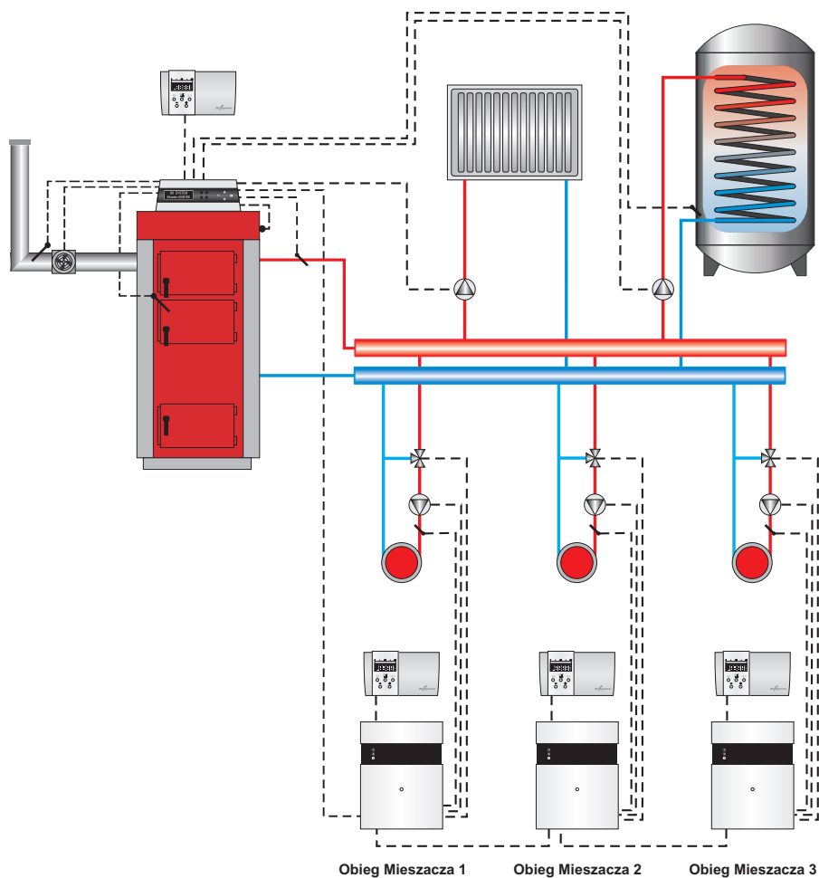
Rys. 7 Przykładowy schemat instalacji z podłączonymi trzema modułami rozszerzającymi DKMZ 1 Obiegu Mieszacza 1 , Obiegu Mieszacza 2 i Obiegu Mieszacza 3 .
