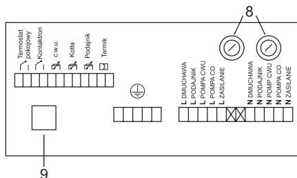
Rys.2 Schemat złączy na tylnej ścianie regulatora w wersji MASTER 300 ver.1 oraz MASTER 300 ver. 3.
