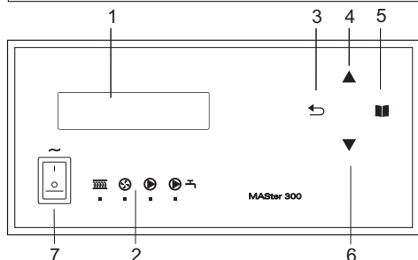
Rys.1 Opis panelu przedniego regulatora
