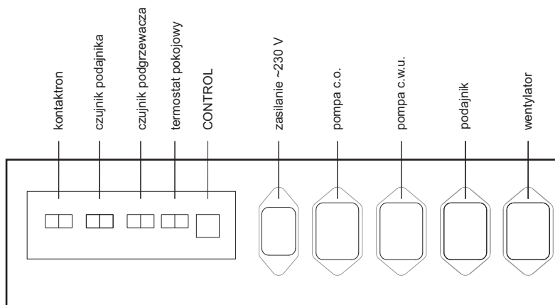
Rys. 6 Schemat elektryczny podłączeń do konsoli przyłączeniowej dla MASTER 300 ver. 2.
