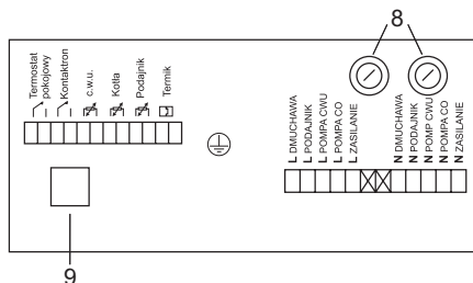
Rys. 3 Schemat złączy na tylnej ścianie regulatora w wersji MASTER 300 ver. 2.
