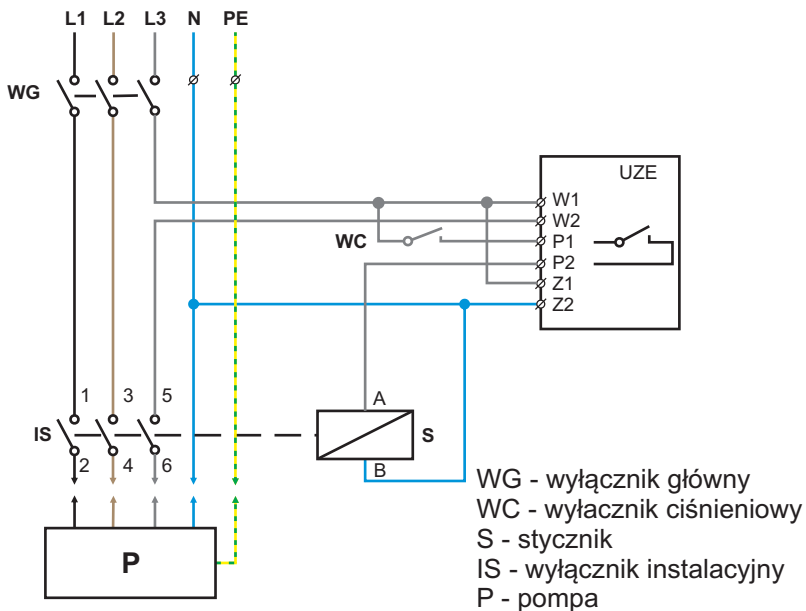
Rys. 3 Schemat połączeń układu z pompą o zasilaniu 3x400V i wyłącznikiem ciśnieniowym
